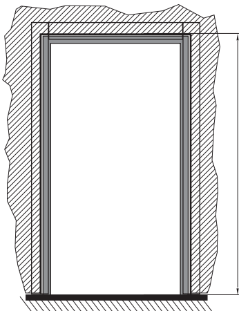
גובה משקוף סטנדרט: 210 ס"מ מקסימלי: 225 ס"מ
